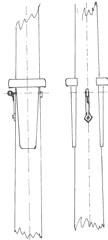
Kranbolzen 1:8
